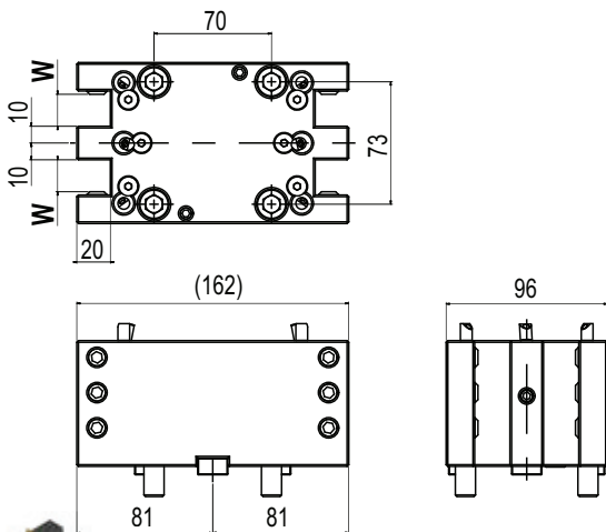
TIPO - TYPE Stelo quadro rad. quadruplo 4 RD face and cutting holder
