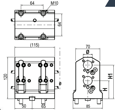
TIPO - TYPE Portabareno doppio Double boaring bar holder
