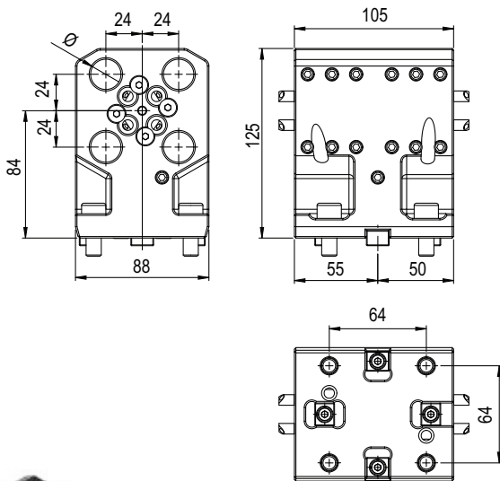
TIPO - TYPE Portabareno 4 posizioni 4 pos. Boring bar tool holder
