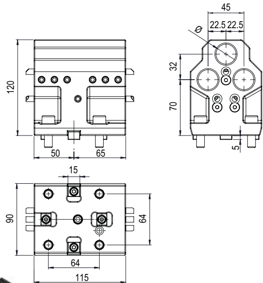
TIPO - TYPE Portabareno 3 posizioni 3 pos. Boring bar tool holder
